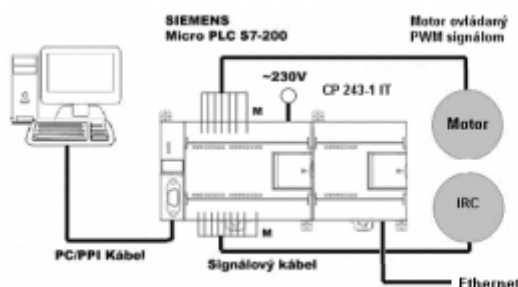
Obr.1. Schéma zapojenia
