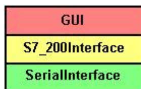
Obr. 6. Architektúra programu
